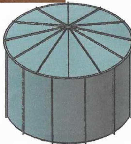
Primer sestavljanja rezervoarjev večjih dimenzij
