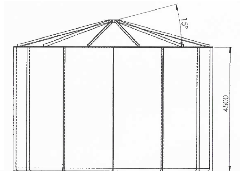
Primer sestavljanja rezervoarjev večjih dimenzij
