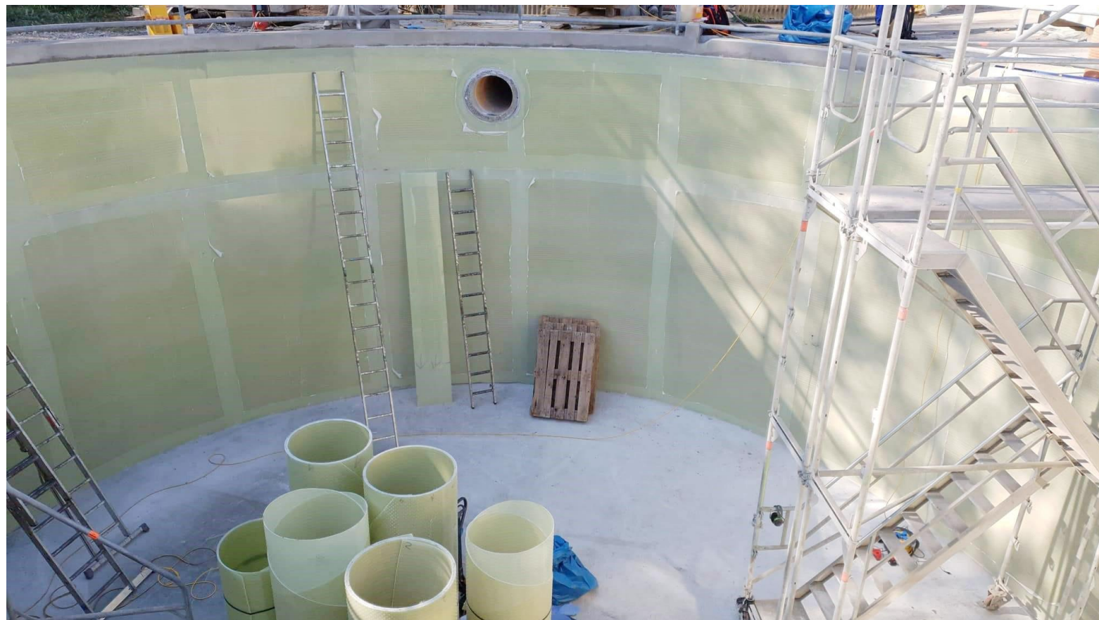
Stari dotrajani betonski rezervoarji
